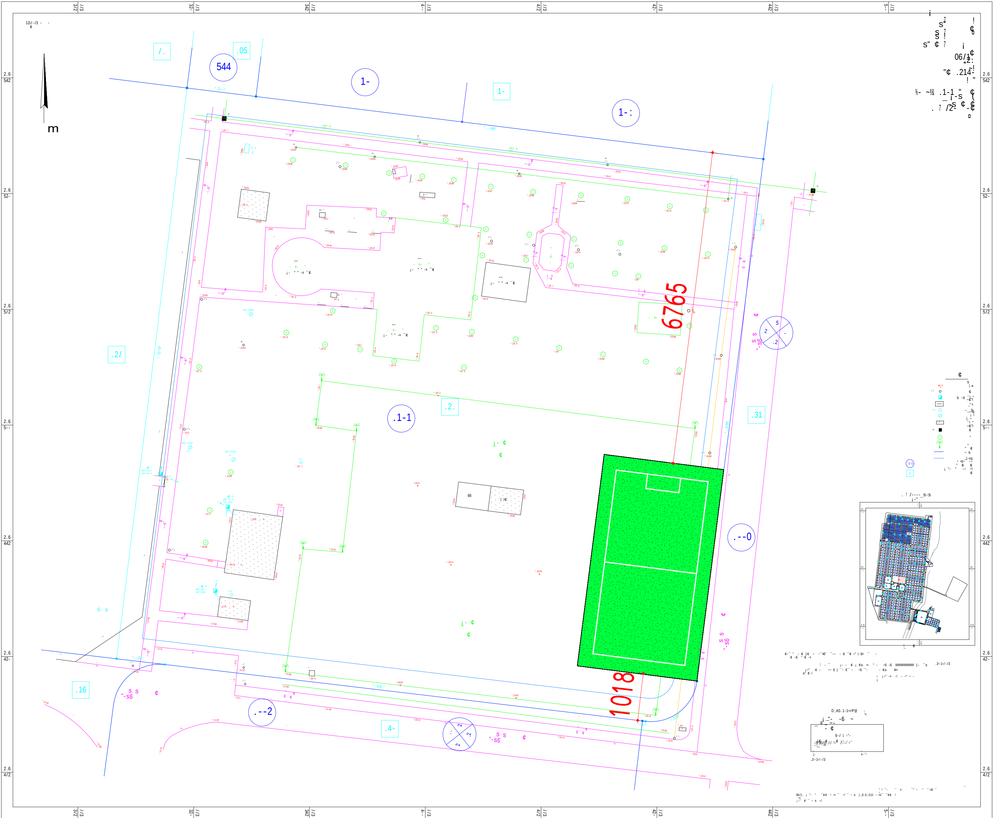
1 העמדה מגרש כדורגל/חצבה 1 : 500
